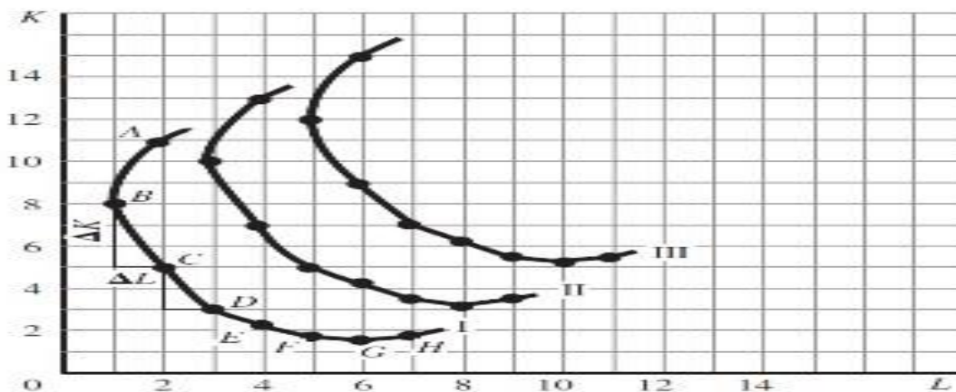
Figura 4. Curvas de isocuantas de una producción
