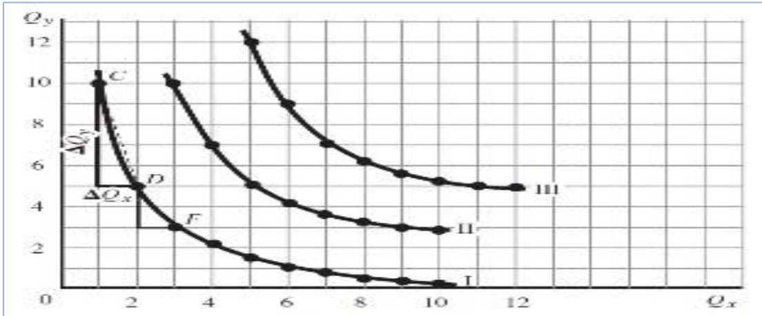
Figura 3. Curvas de indiferencia para un consumidor
