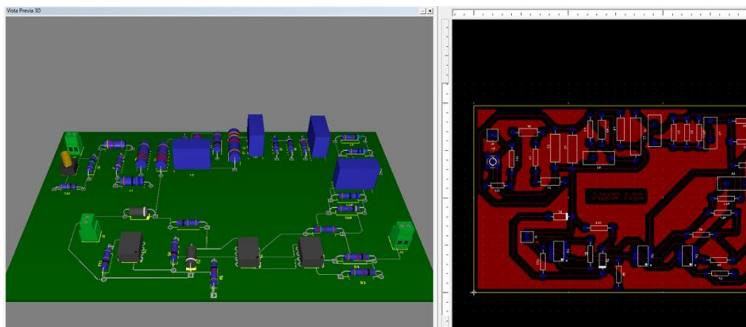
Figura 2: Diseño de la placa PCB del receptor VLF.
