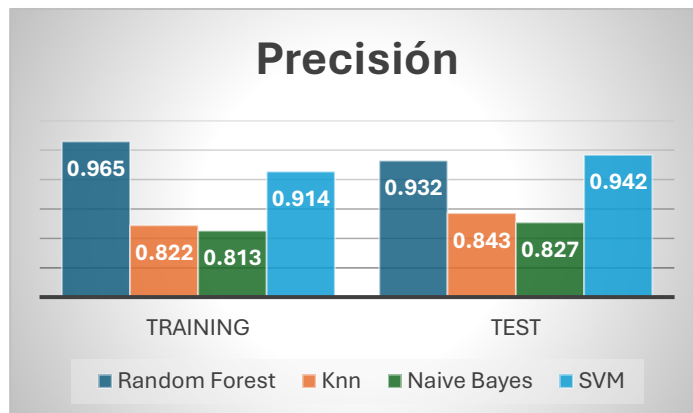
Figura 3. Reporte de clasificación.
