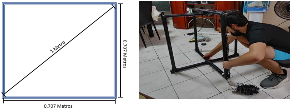
Figura 1: Diseño e implementación de antena de cuadro basados en dos loops.
