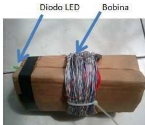
Figura 4 Disposición de la Bobina del Prototipo
