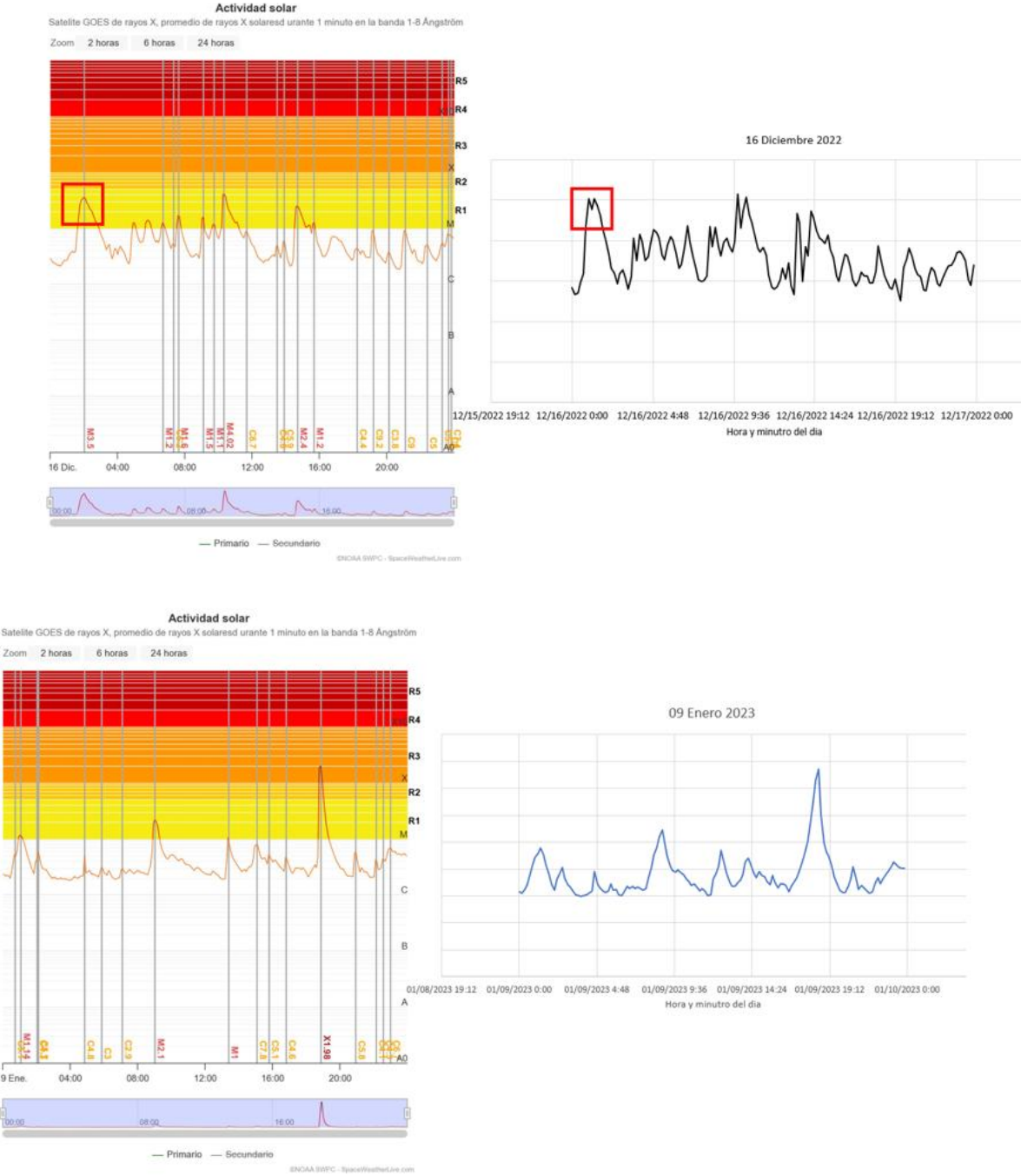
Figura 6a: Eventos de Llamadas Solares proporcionado por el sitio SoHo (Izquierda) y los capturados por la unidad de recepción VLF desarrollada (derecha) del 16 de diciembre de 2022 y 9 de enero de 2023.
