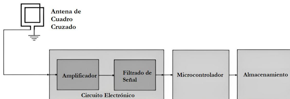
Figura 3: Diagrama bloque simplificado de la unidad capturadora de datos de las llamadas solares.
