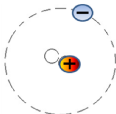
Figura 1 Estructura Atómica (Ernest Rutherford, 1911)
