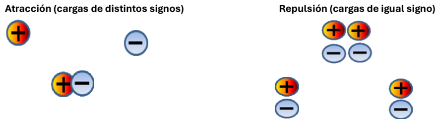
Figura 2. Proceso de Atracción y Repulsión de la Cargas. (Coulomb de 1785)
