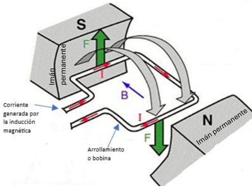
Figura 5 Diagrama pictórico, funcionamiento del prototipo
