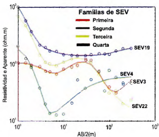
Fig. 8. Modelos 1D ajustados com inversão.
