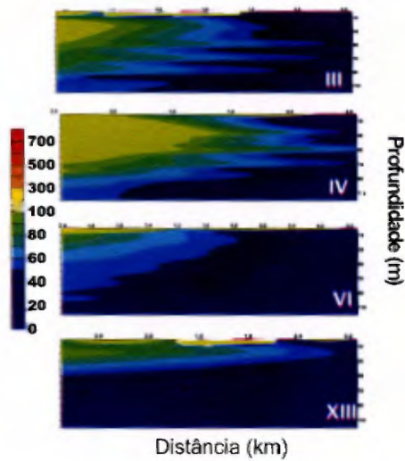
Fig. 9. Seções geolétricas dos perfis III, IV, VI e XIII no sentido E-W.
