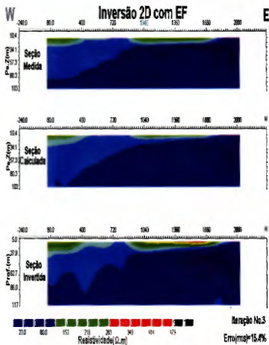
Fig. 11. Inversão do Perfil XIII com elementos finitos.
